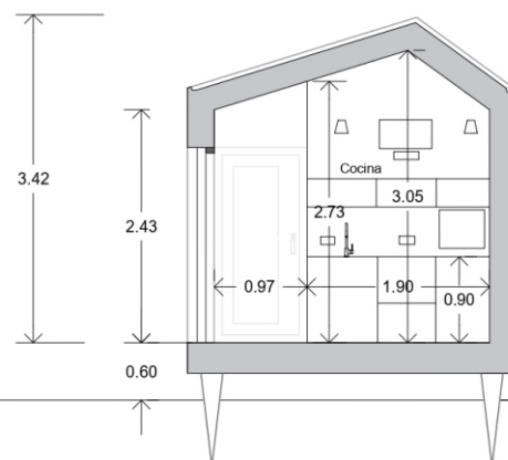
CORTE 3 SECTOR COCINA
