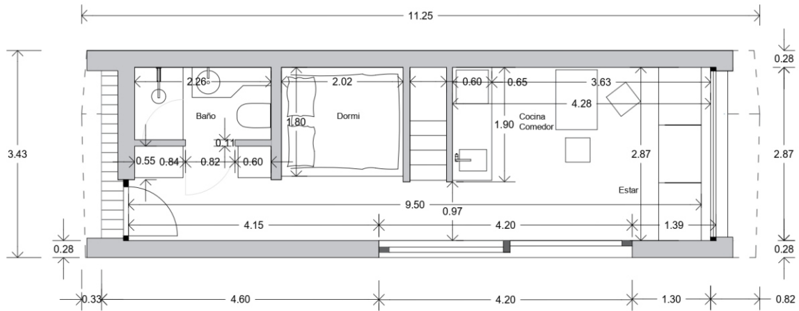
CORTES CON ALTURAS INTERIORES CORTE 1 LONGITUDINAL
