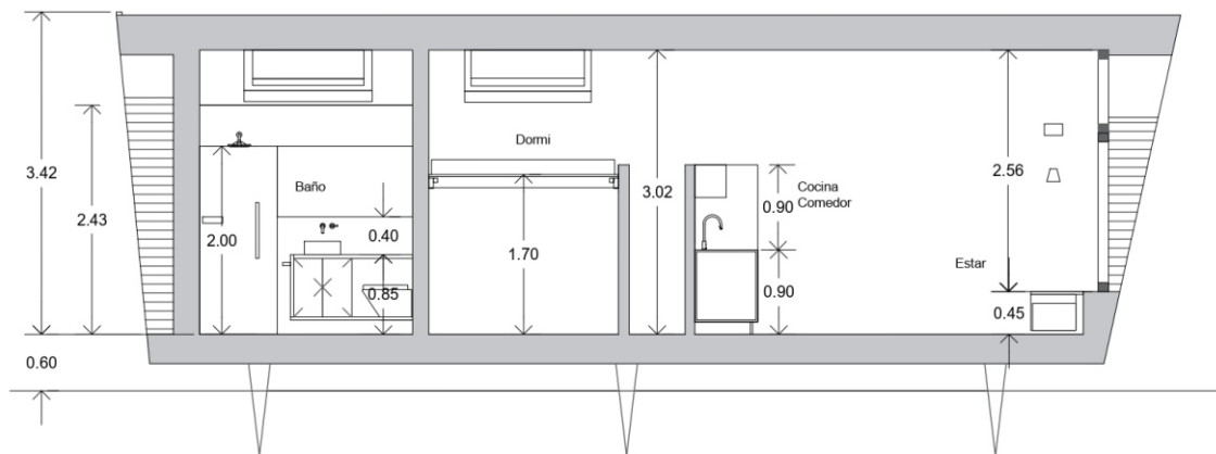
CORTE 2 SECTOR BAÑO
