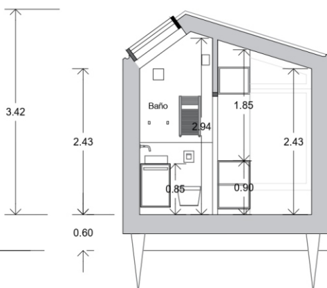
CORTE 2 SECTOR BAÑO
